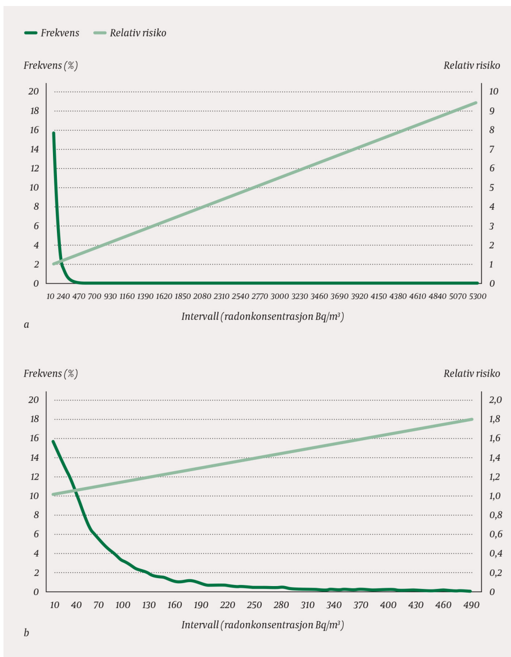
Figur 1 a) Frekvensfordeling av ulike radonkonsentrasjoner i norske boliger (venstre akse, mørkegrønn kurve) og beregnet relativ risiko (RR) for lungkreft (høyre akse, lysegrønn kurve) som funksjon av radonkonsentrasjon i norske boliger (x-aksen) i den landsomfattende kartleggingen i 2000-01 (3, 10) – hele datasettet (når vi antar lineær risikoøkning også over 800 Bq/m 3 ). b) Frekvensfordeling av ulike radonkonsentrasjoner i norske boliger (venstre akse, mørkegrønn kurve) og beregnet relativ risiko (RR) for lungkreft (høyre akse, lysegrønn kurve) som funksjon av radonkonsentrasjon i norske boliger (x-aksen) i den landsomfattende kartleggingen i 2000-01 (3, 10) – kun boliger med radonkonsentrasjon 0–500 Bq/m 3
